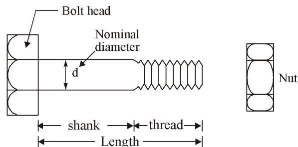
Fig. : Bolt and Nut
