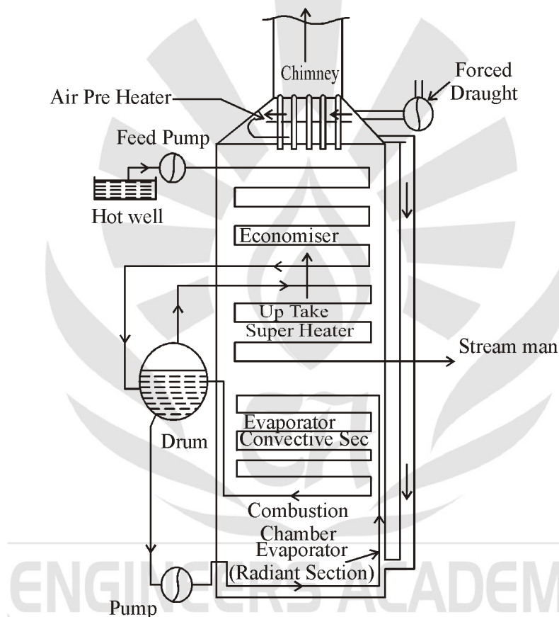
Fig. : Lamont boiler
